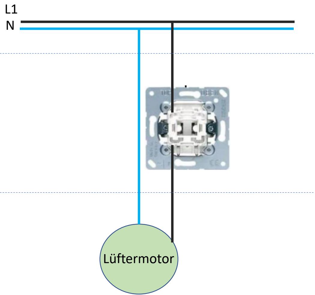
Standardfall Kabel mit N und L über Schalter zum Motor
